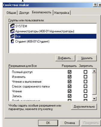
Рис.6. Всем пользователям даны все права
