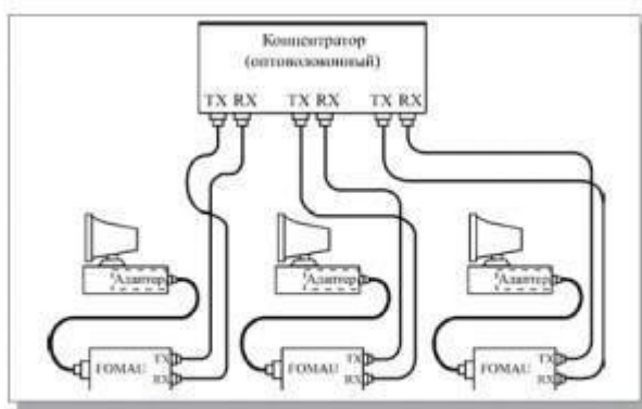
Рисунок 7 – Соединение адаптера и концентратора в 10BASE-FL
